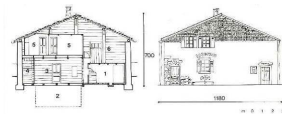
Coupe et façade d'une maison de Vallorcine, au Couteray : 1/ écurie, 2/ cave, 3/ pèle, 4/ couloir, 5/ chambre haute, 6/ grange. Source : L'architecture rurale française, Savoie. Henri Raulin, ed Berger-Levrault 1977.
