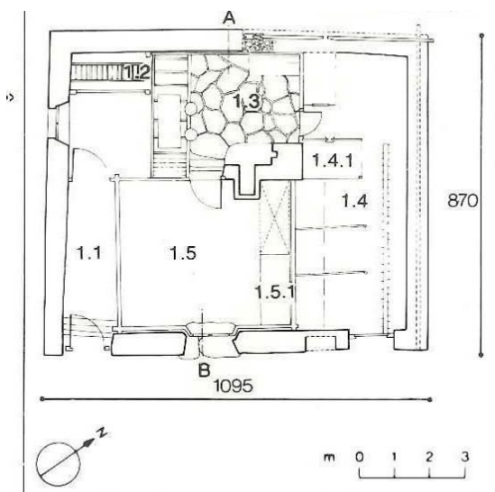
Plan d'une maison de Vallorcine : 1.1/ couloir « étra », 1.2/ montée à la grange, 3/ cuisine « outa », 1.4/ écurie, 1.4.1 loge à cochon, 1.5/ chambre « pèle », 1.5.1/ lit. Source : L'architecture rurale française, Savoie. Henri Raulin, ed Berger-Levrault 1977.
