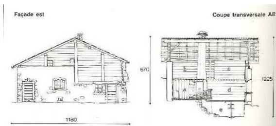
Façade et coupe d'une maison de Vallorcine au Couteray : a/ cuisine « outa », b/ grange, c/ chambre haute, d/ pèle, e/ cave. Source : L'architecture rurale française, Savoie. Henri Raulin, ed Berger-Levrault 1977.
